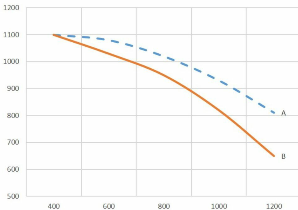
A: Fan total Pressure B: Fan Static Pressure X: m³/h Y: Pa
